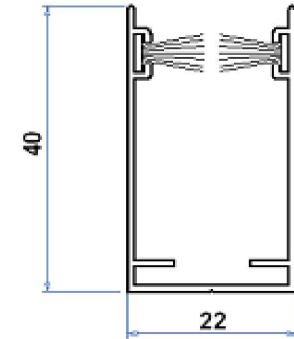
Боковая направляющая, тип 1
