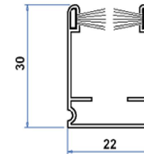
Боковая направляющая, тип 2
