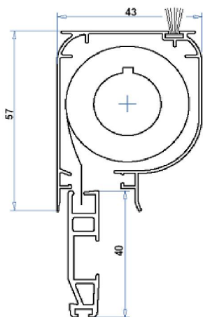
Сечение короба с валом, сеткой и тяговой планкой
