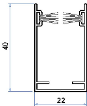
Верхняя направляющая, тип 1
