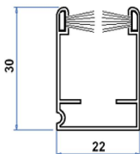
Верхняя направляющая, тип 2
