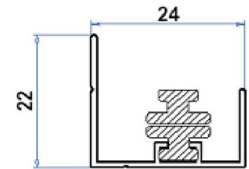
Боковой профиль с магнитом
