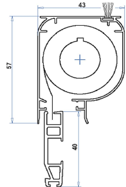
Короб с валом, сеткой и тяговой планкой
